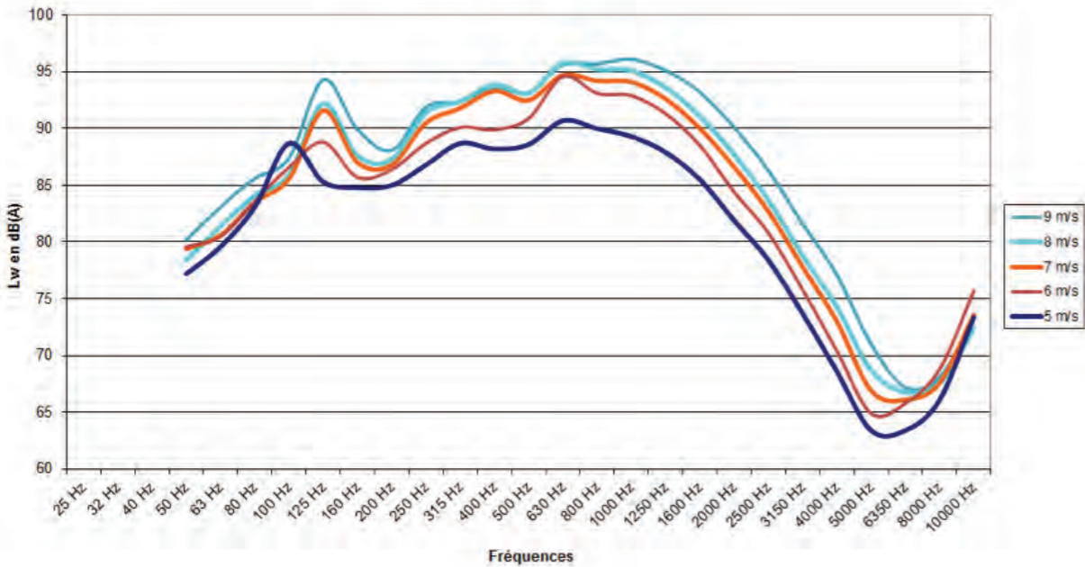
FIGURE 186 : SPECTRES D'ÉMISSION ENERCON E92
