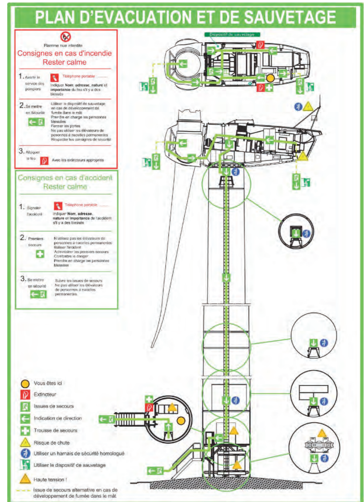
FIGURE 189 : EXEMPLE DE PLAN D'ÉVACUATION DE L'ÉOLIENNE
