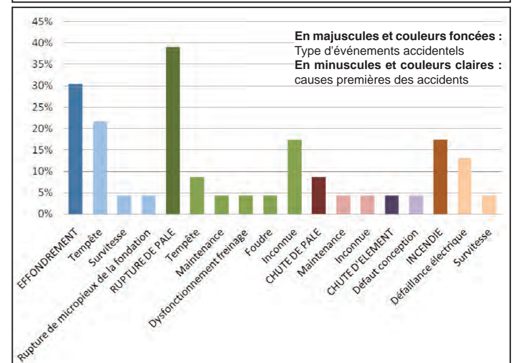
FIGURE 160 : RÉPARTITION DES ÉVÉNEMENTS ACCIDENTELS ET DE LEURS CAUSES PREMIÈRES SUR LE PARC D'AÉROGÉNÉRATEURS FRANÇAIS ENTRE 2000 ET 2011
