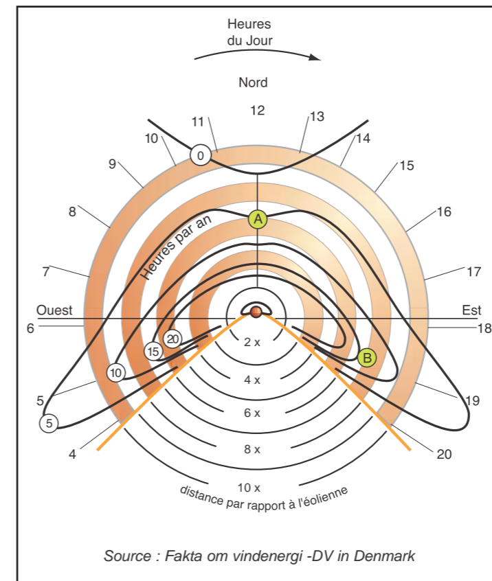
FIGURE 131 : PROJECTION DES OMBRES EN FONCTION DES HEURES DE LA JOURNÉE ET DE LA HAUTEUR DU MAT
