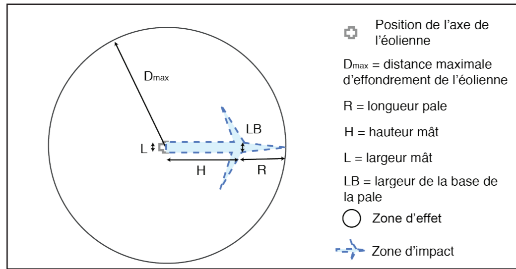
FIGURE 166 : SCHÉMATISATION DU SCÉNARIO EFFONDREMENT DE L'ÉOLIENNE
