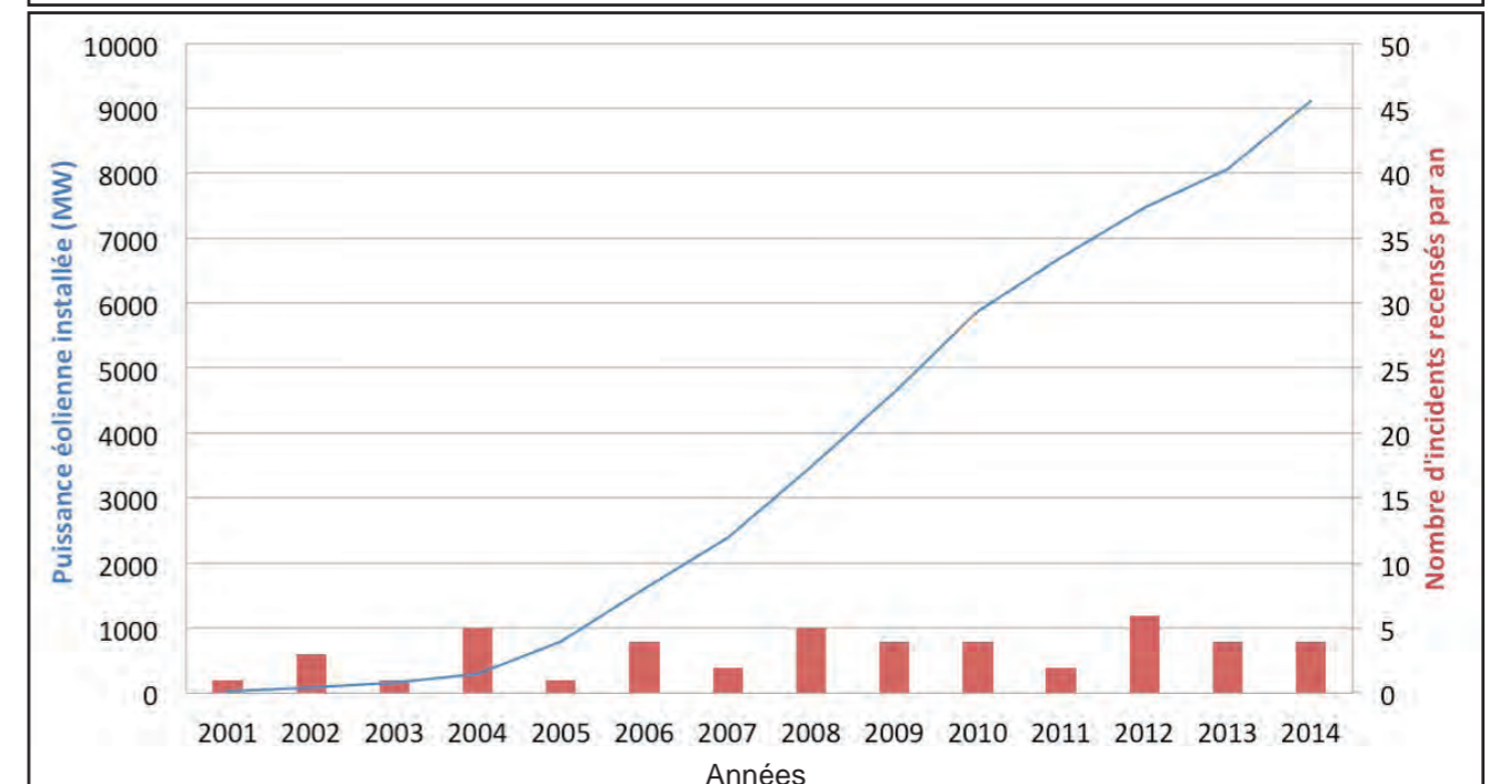
FIGURE 162 : MISE EN PARALLÈLE DE L'ÉVOLUTION DU PARC ÉOLIEN FRANÇAIS ET ÉVOLUTION DU NOMBRE D'INCIDENTS RECENSÉS CHAQUE ANNÉE
