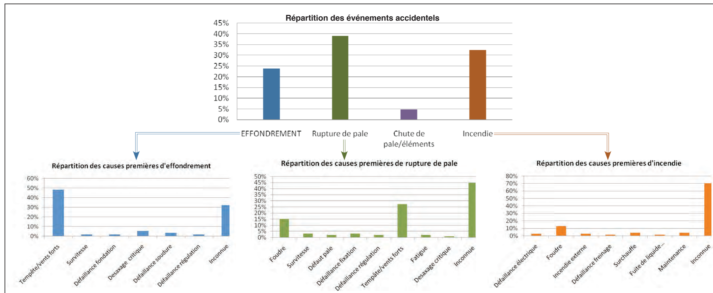
FIGURE 161 : RÉPARTITION DES ÉVÉNEMENTS ACCIDENTELS ET DE LEURS CAUSES PREMIÈRES SUR LE PARC D'AÉROGÉNÉRATEURS MONDIAL ENTRE 2000 ET 2011
