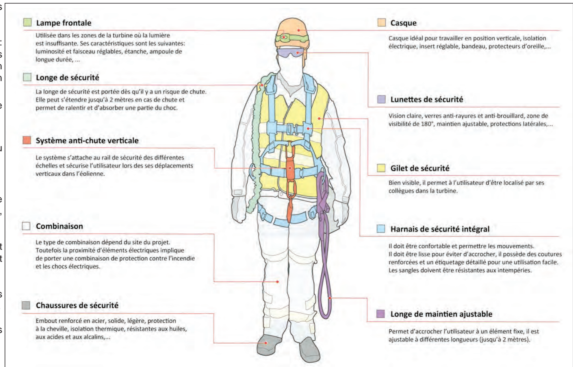
FIGURE 188 : LES DIFFÉRENTS EPI POUR LA MAINTENANCE ÉOLIENNE
